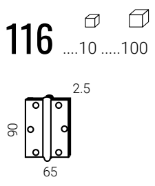
Bisagras canto cuadrado Straight corner flat hinge
